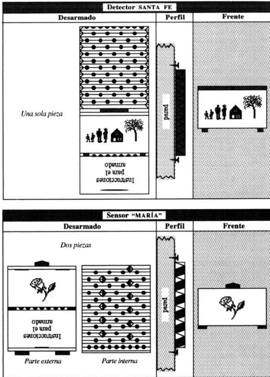
Fig. 1.- Diferencias de diseño entre ambos detectores
